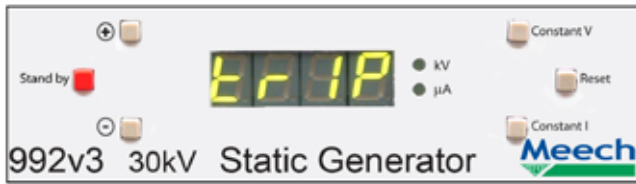
Display des 992v3 in der Trip-Funktion
